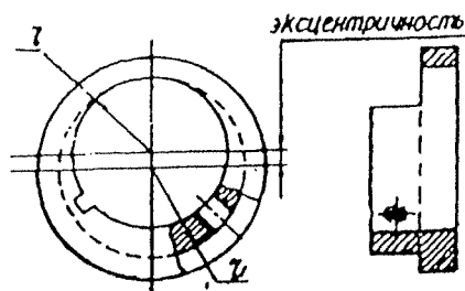
Рис.7 Эксцентрическое кольцо.
