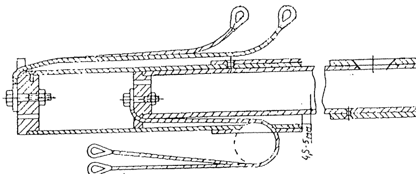
Рис.5 Сборка подвижных коленей мачты.
