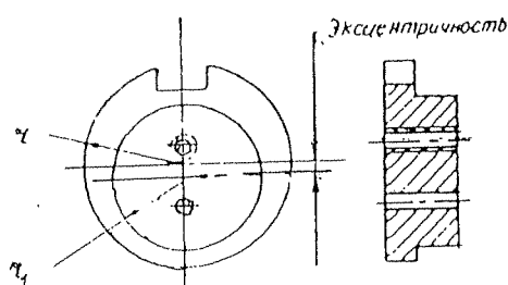
Рис.6 Эксцентрическое основание.
